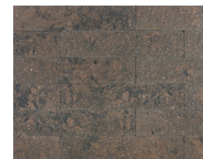
bronzite
